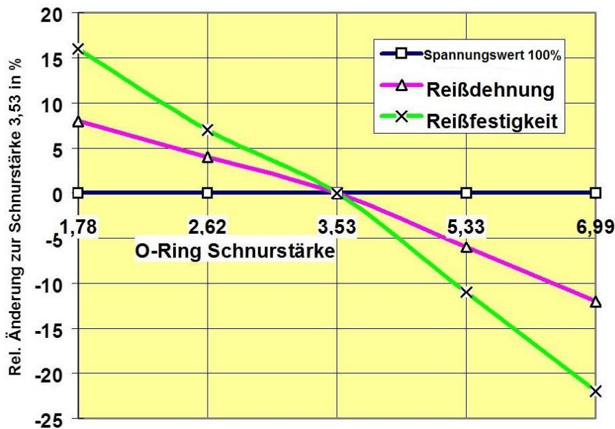
Abb. 8: Relative Änderung des Spannungswertes \sigma 100%, der Reißdehnung und Reißfestigkeit in Abhängigkeit von der Schnurstärke von O-Ringen 28 .
