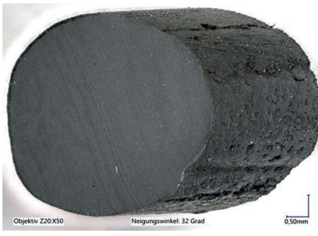
10 Oberflächenbeschädigung eines O-Rings durch harte Kavitation an einer nassen Zylinderlaufbuchse
