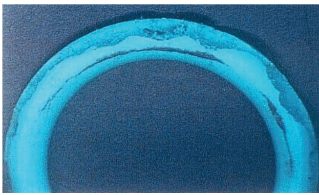
11 Geschädigter O-Ring durch Spaltextrusion: Die Ausbrüche ähneln dem Schadensbild einer Explosiven Dekompression
