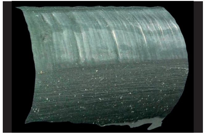
12 Geschädigte O-Ring Oberfläche durch Blow-by Effekte infolge harter Druckstöße: Dieses Schadensbild kann einer Strömungserosion ähneln
