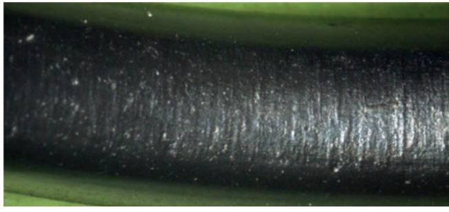
09 Erosionsschäden (parallele Riefen in Axialrichtung) an einem O-Ring
